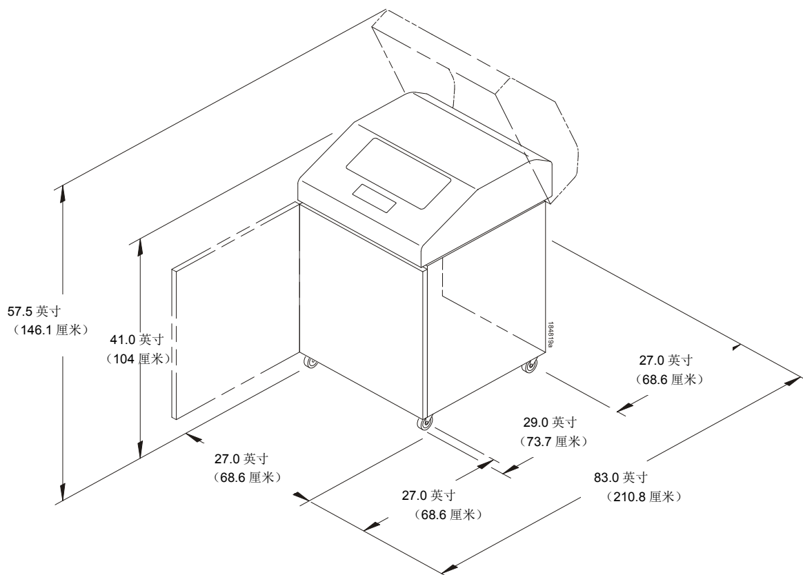
图2. 柜式打印机
