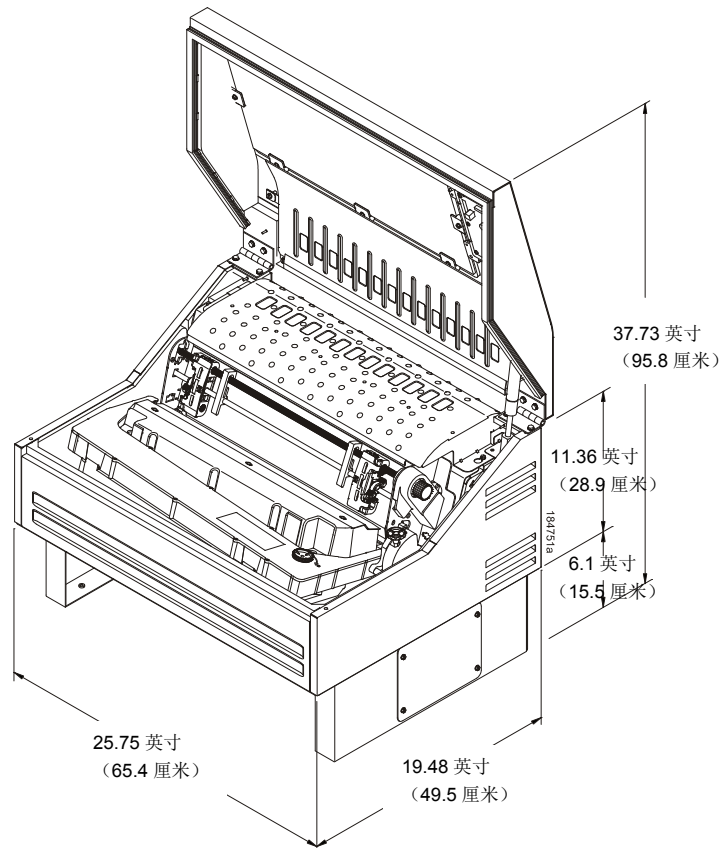
图1 台式打印机
