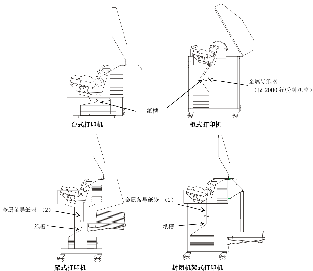
图8. 纸槽位置
