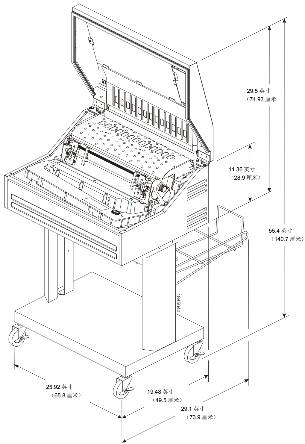
图4. 架式打印机
