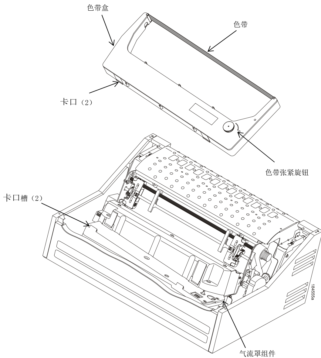
图21. 安装色带盒
